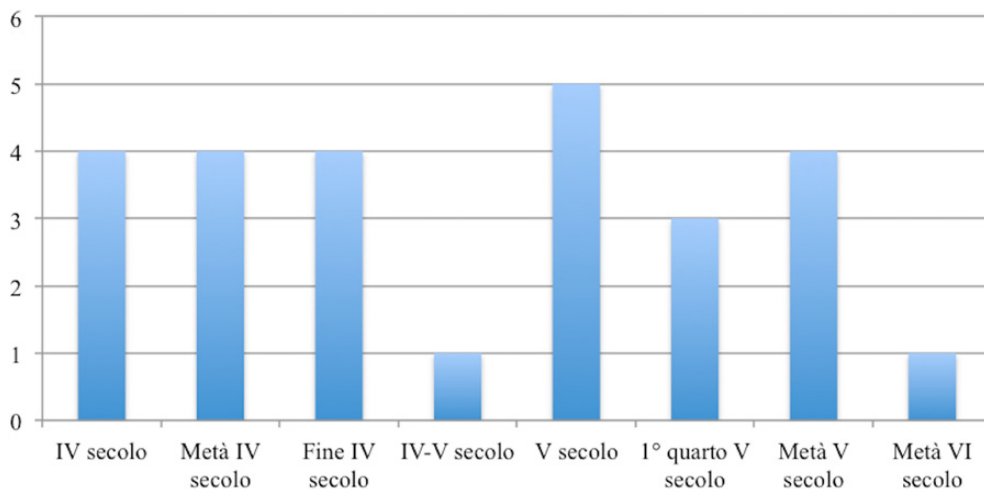
Fig. 2. Datazione dei mosaici funerari in Hispania.
