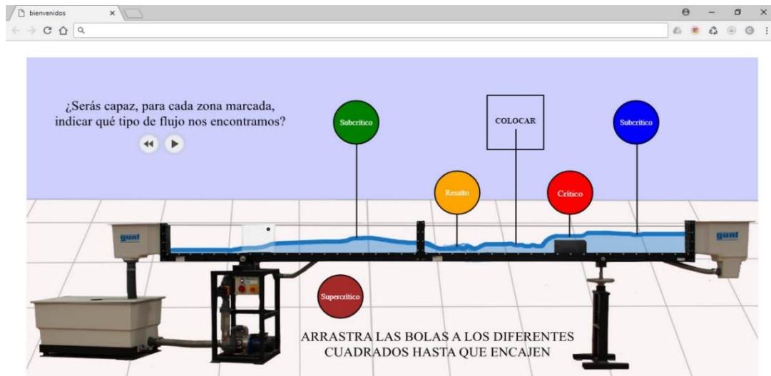
FIGURA 6. Distintos tipos de flujo en el canal
