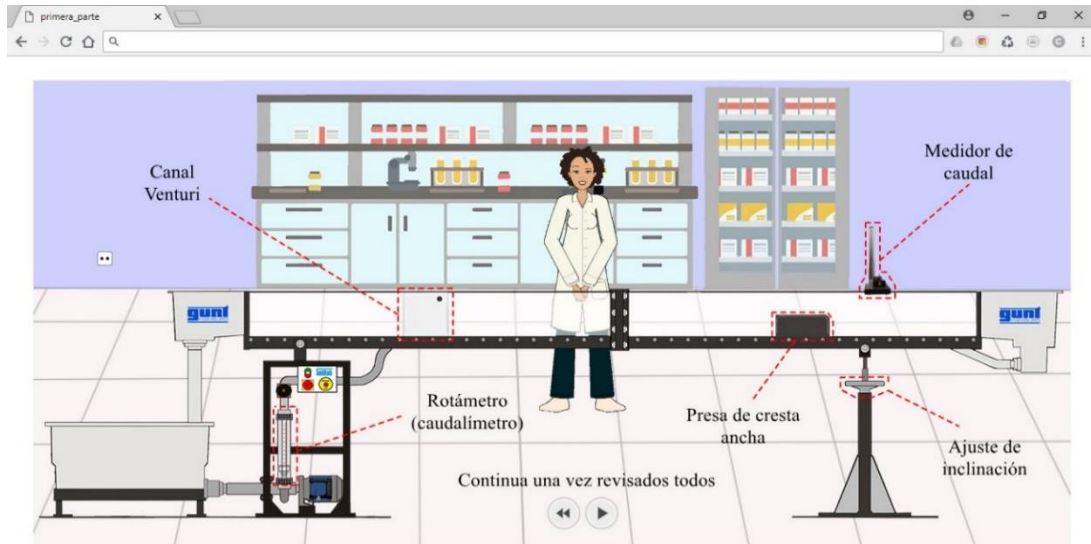
FIGURA 5. Elementos del canal hidrodinámico
