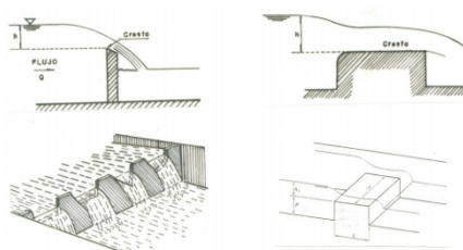
FIGURA 2.1. Flujo a través de vertederos.
