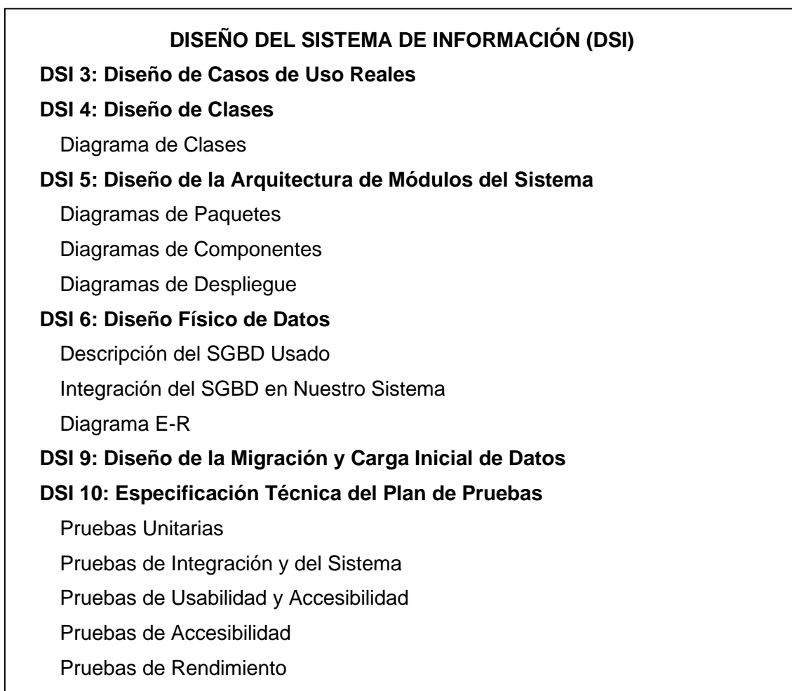
Figura 3. Actividades y tareas de Métrica 3 del proceso DSI incluidos en la plantilla. Fuente: Elaboración propia.
