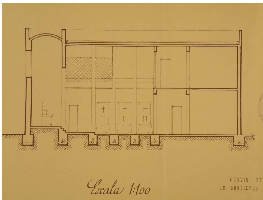
Fig. 8. Casa de Ejercicios Espirituales. Capilla. Detalle de plano sección. Proyecto de reforma. Memoria , octubre de 1955, AHPZa, DPV 33/9.
